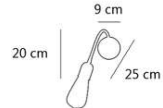
Referencia 10283 Aplique BIRDY Niquel Satinado 1 x E-27
